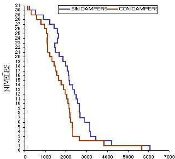
Figura 7 CORTANTES INELASTICAS DE ENTREPISO (t)
