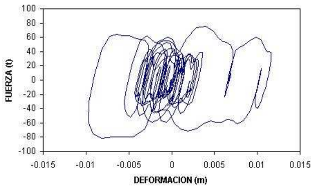
Figura 17 FUERZA-DEFORMACION (NIVEL 10)
