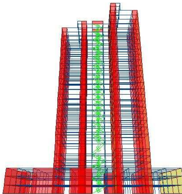
Figura 6 EDIFICIO CON DISIPADORES
