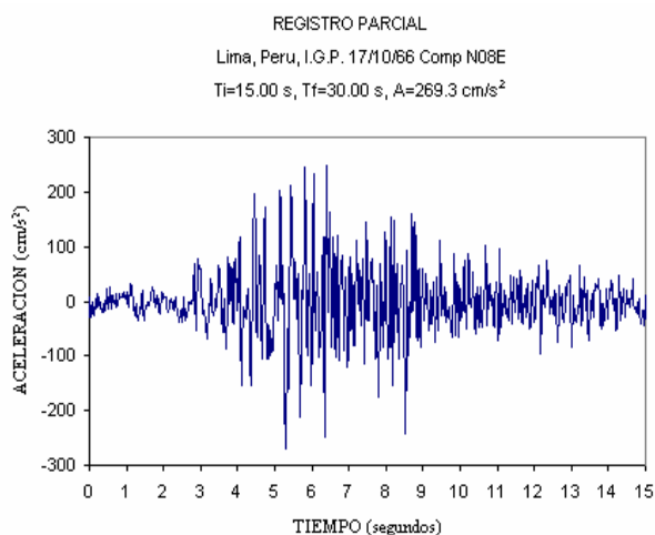
Figura 2 REGISTRO SISMICOPARCIAL
