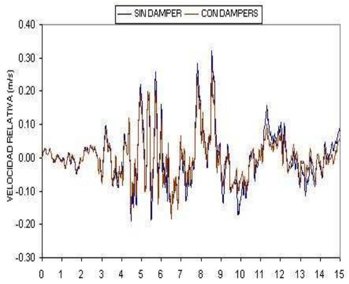
Figura 14 VELOCIDAD EN EL TIEMPO (m/s)
