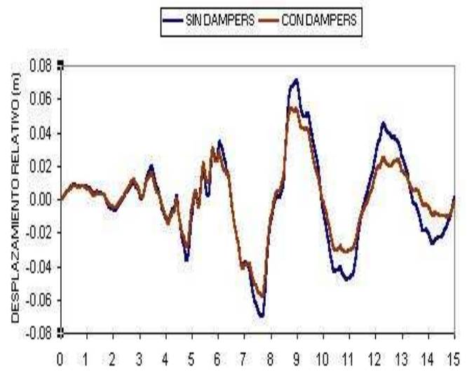
Figura 10 DESPLAZAMIENTO EN EL TIEMPO (s)
