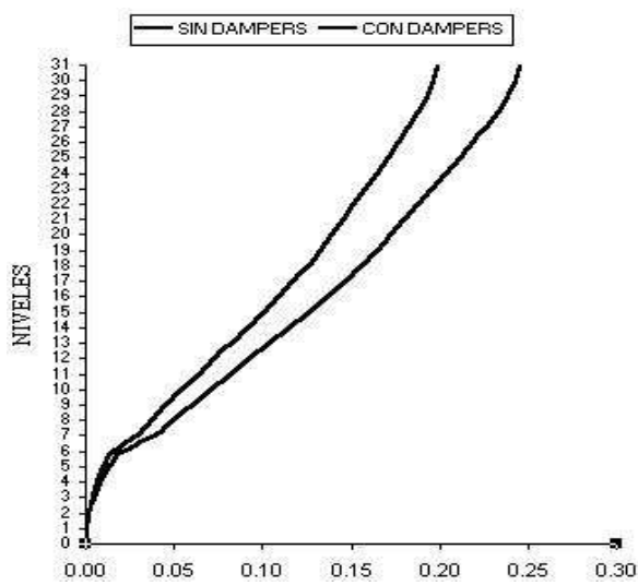
Figura 9 DESPLAZAMIENTO RELATIVO (m)
