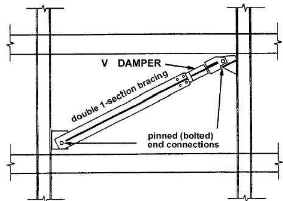
Figura 4 DETALLE DE LA INSTALACION
