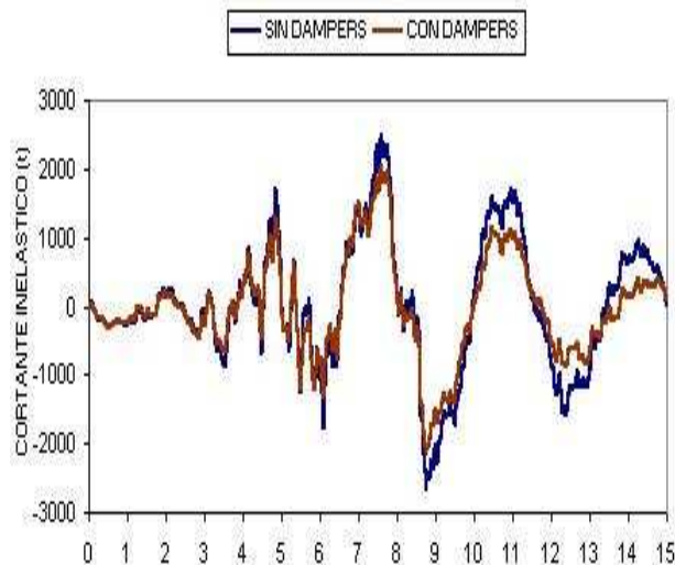
Figura 8 CORTANTE EN EL TIEMPO (s)
