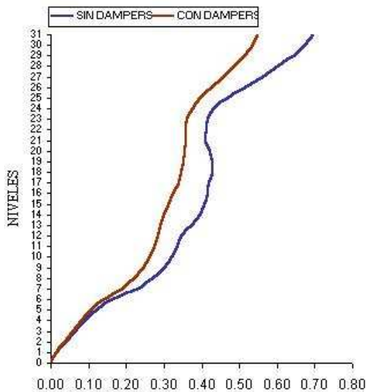
Figura 13 VELOCIDAD RELATIVA (m/s)
