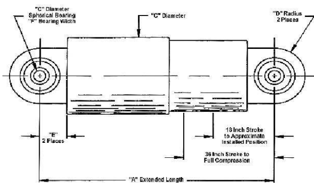
Figura 3 VISTA EXTERIOR DEL DISIPADOR
