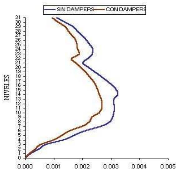
Figura 11 DISTORSIONES EDIFICIO INICIAL
