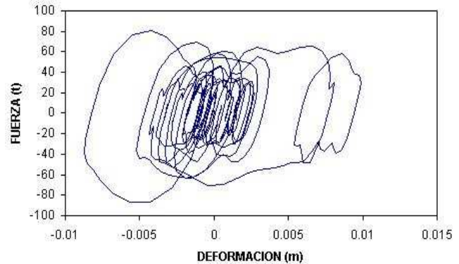
Figura 18 FUERZA-DEFORMACION (NIVEL 20)
