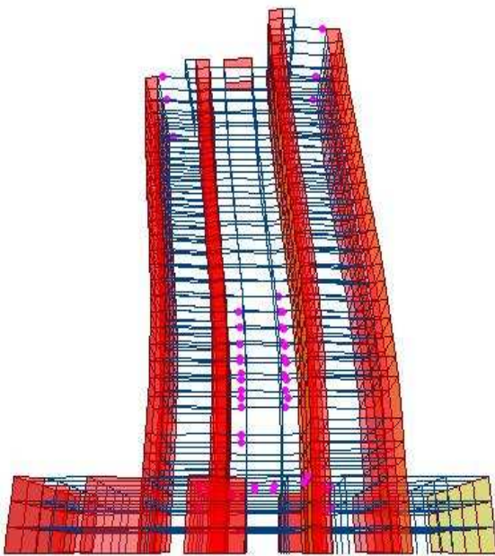
Figura 21 EDIFICIO ROTULADO INICIAL
