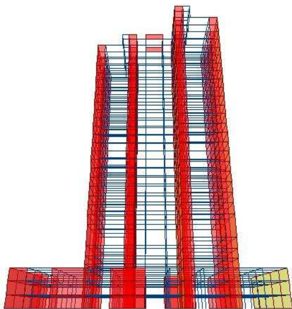
Figura 5 EDIFICIO INICIAL
