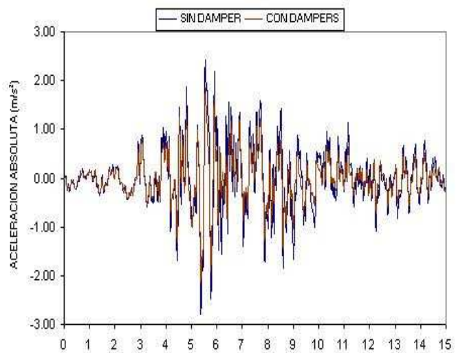
Figura 16 ACELERACION EN EL TIEMPO (m/s 2 )
