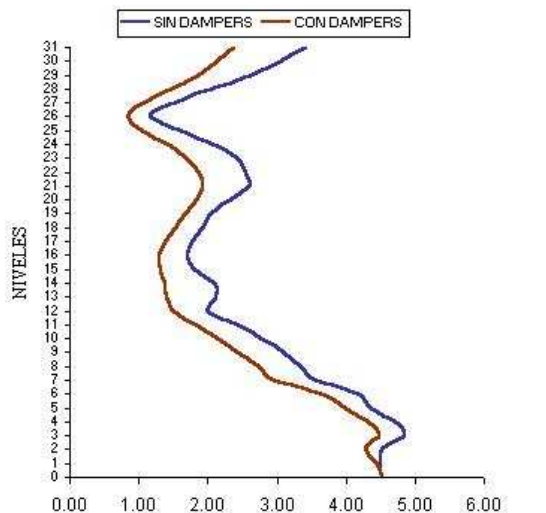
Figura 15 ACELERACION ABSOLUTA (m/s 2 )
