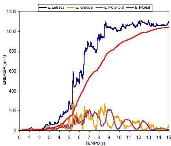
Figura 19 ENERGÍA EDIFICIO CON DISIPADORES
