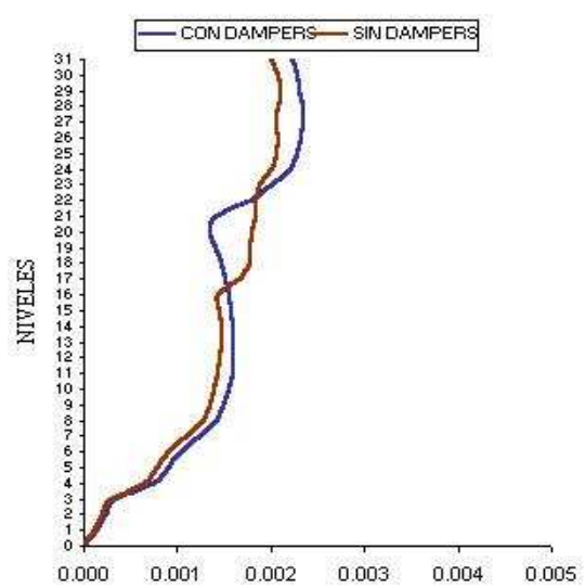
Figura 12 DISTORSIONES ON DISIPADORES
